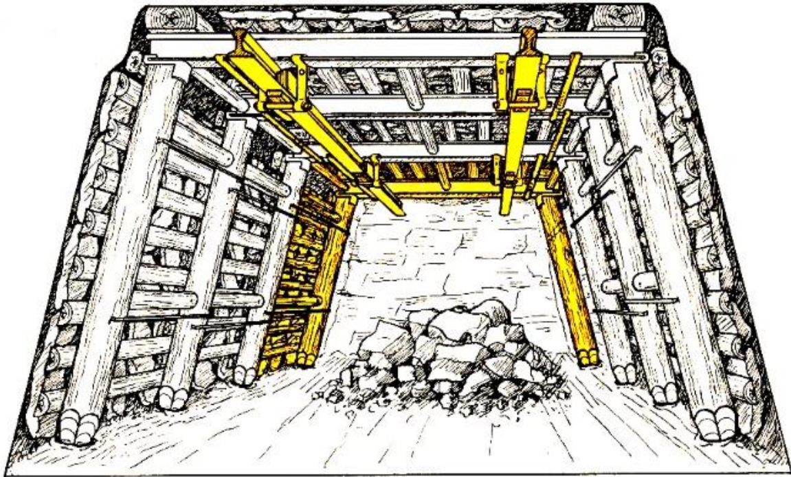
Stand der Arbeit bei den Arbeitsstufen 13 und 14
