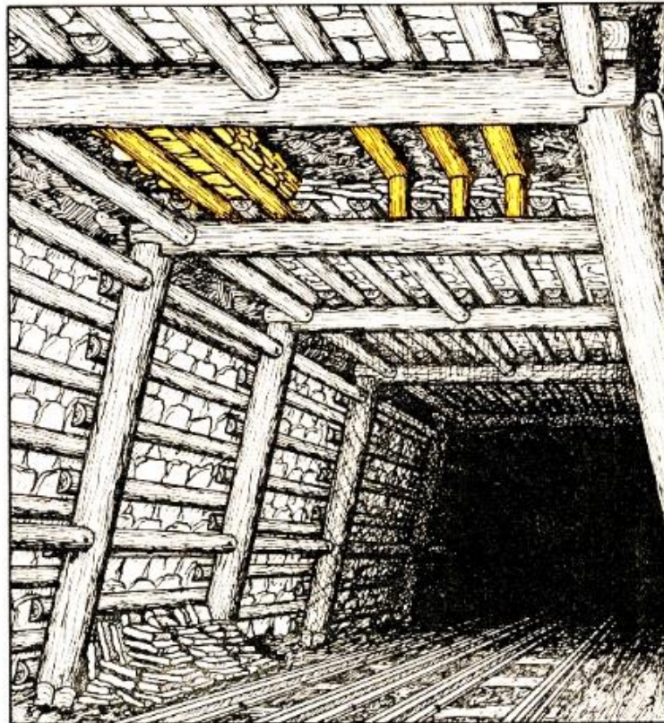
Erneuern des Firstenverzuges
