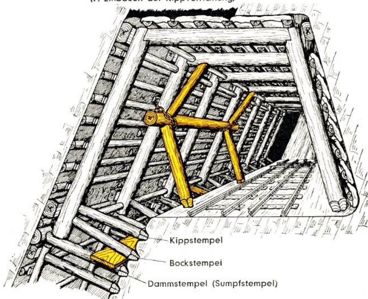
Stand der Arbeit nach Arbeitsstufe 6
