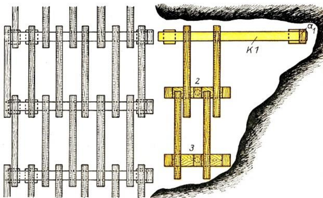
Stand der Arbeit nach Arbeitsstufe 8
