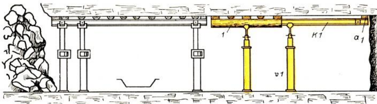
Stand der Arbeit nach Arbeitsstufe 5
