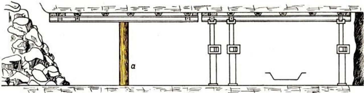
Stand der Arbeit nach Arbeitsstufe 6
