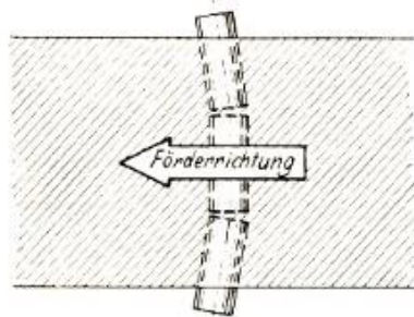
Arbeitsstufe 8: Richtige Lage der Oberbandrollen
