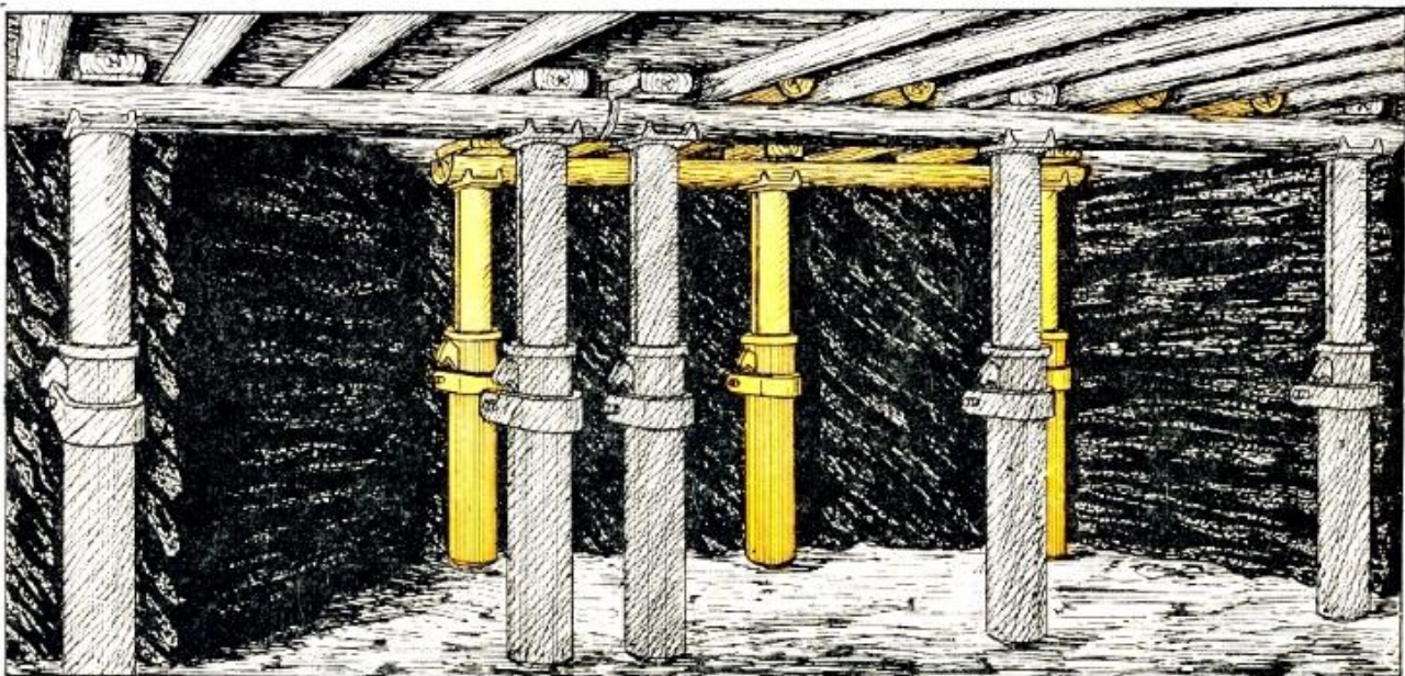
Stand der Arbeit nach Arbeitsstufe 13
