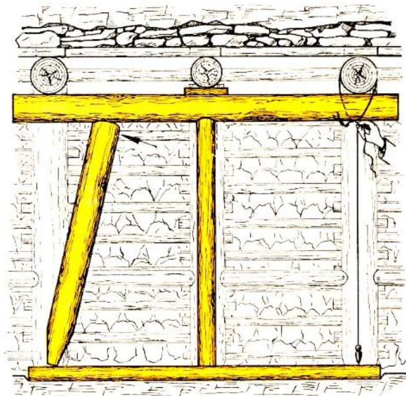
Stand der Arbeit bei Arbeitsstufe 7
