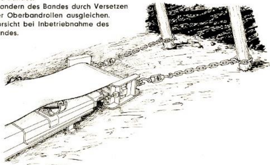
Umkehr- und Spannstation
