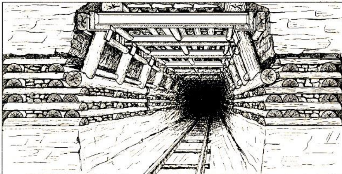
Gemischter Türstock auf Bergekästen
