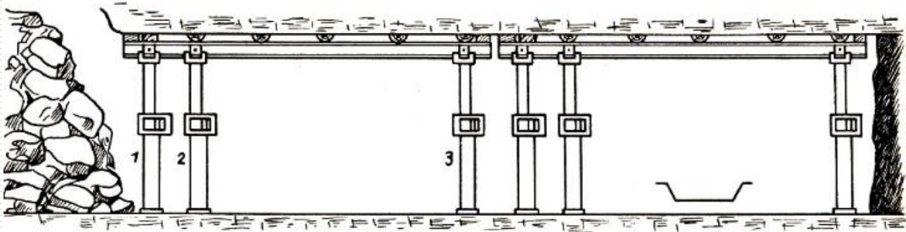
Stand der Arbeit zu Beginn der Raubschicht
