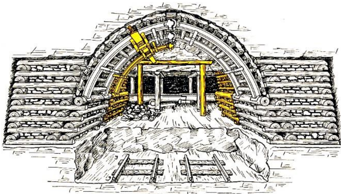
Stand der Arbeit nach Arbeitsstufe 7
