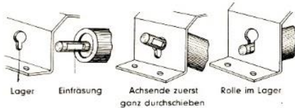
Arbeitsstufe 9: Einlegen der Unterbandrollen
