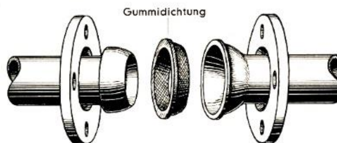
Kugelflanschverbindung
