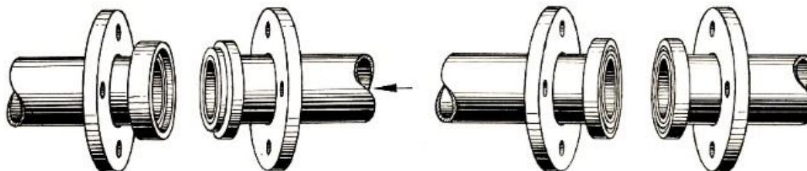
Flanschverbindung mit Vor- und Rücksprung
