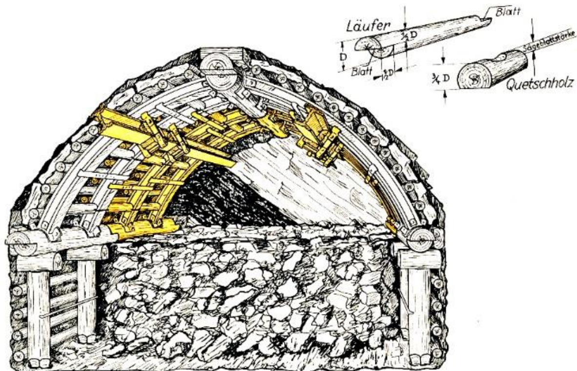
Stand der Arbeit nach Arbeitsstufe 7
