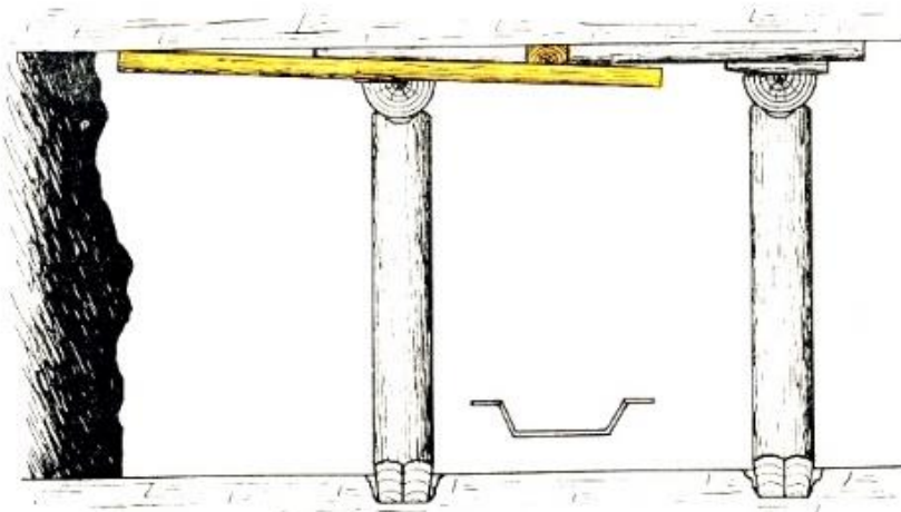
Spitze 1 nach Arbeitsstufe 5
