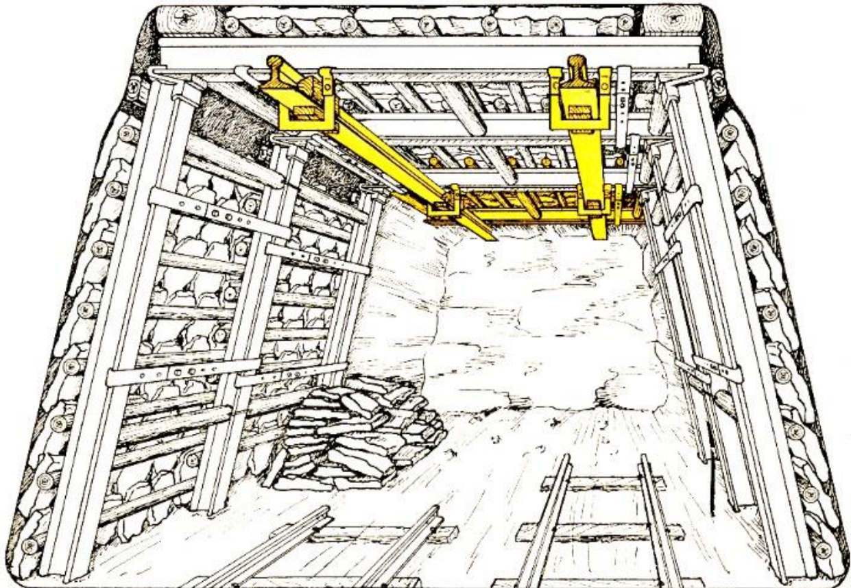
Stand der Arbeit nach Arbeitsstufe 8
