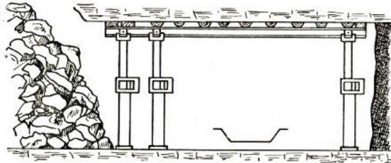
Stand der Arbeit bei Beginn der Kohlenschicht.
