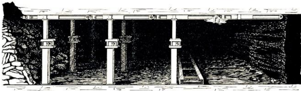
Stand der Arbeit nach Arbeitsstufe 5
