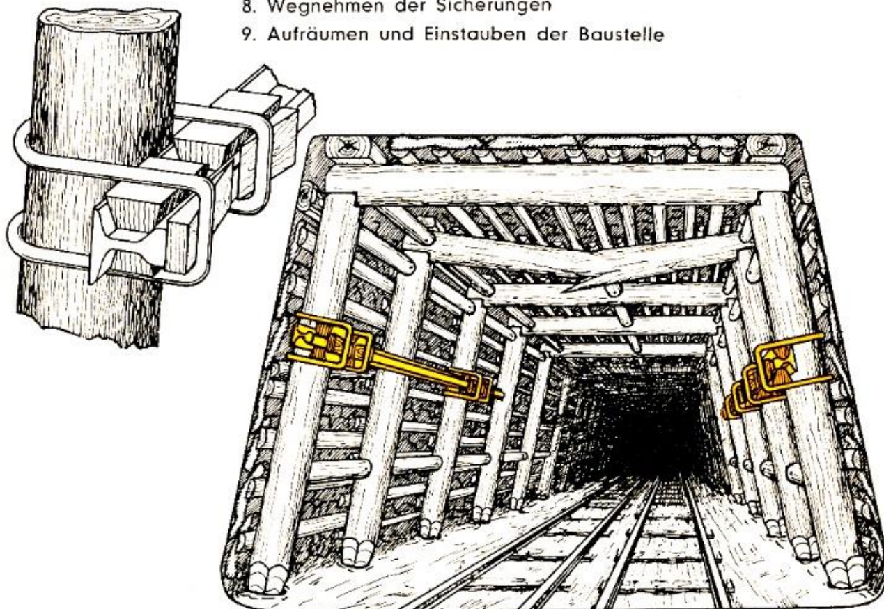
Stand der Arbeit nach Arbeitsstufe 1
