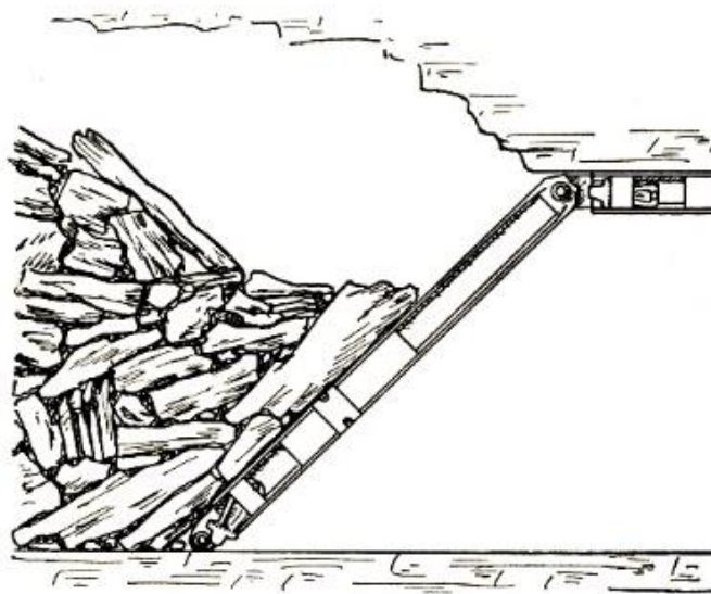
Stand der Arbeit nach Arbeitsstufe 2
