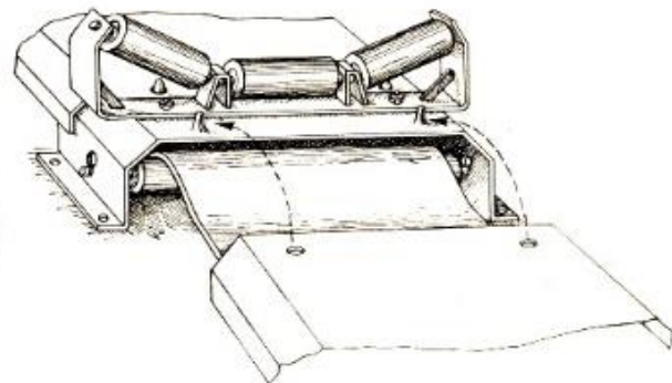
Arbeitsstufe 10: Auflegen der Abdeckbleche
