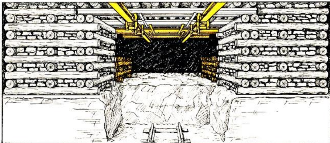
Stand der Arbeit bei Arbeitsstufe 7
