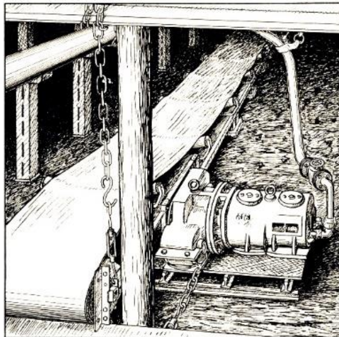
Antrieb
