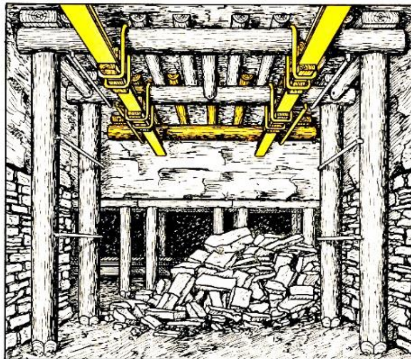
Stand der Arbeit nach Arbeitsstufe 6
