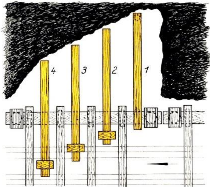
Stand der Arbeit nach Arbeitsstufe 9
