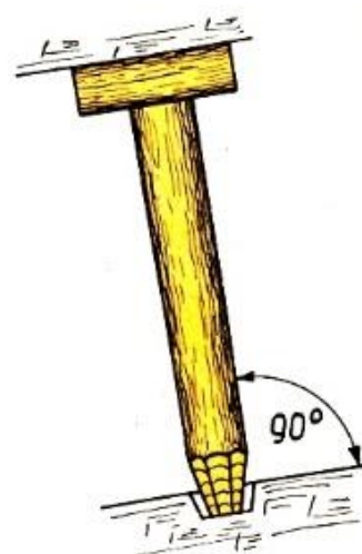
Richtig gesetzter Stempel
