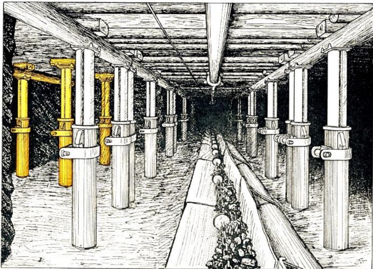
Stand der Arbeit nach Arbeitsstufe 8
